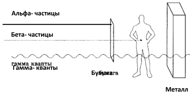
Сурет 3.3. Әр түрлі сәулеленудің ену қабілетінің схемалық бейнесі
