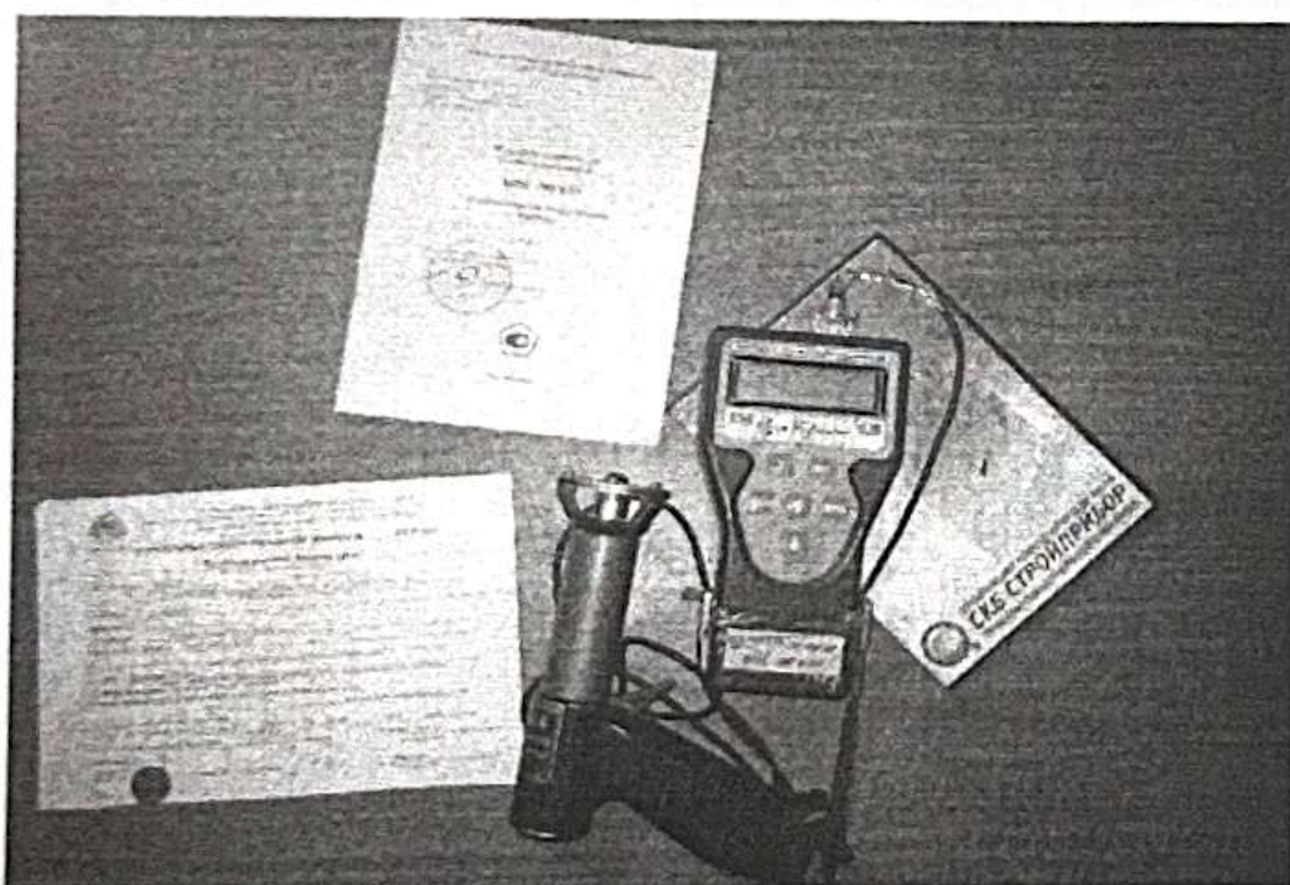
Электронный измеритель защитного слоя бетона «ИЗС-10Ц»
