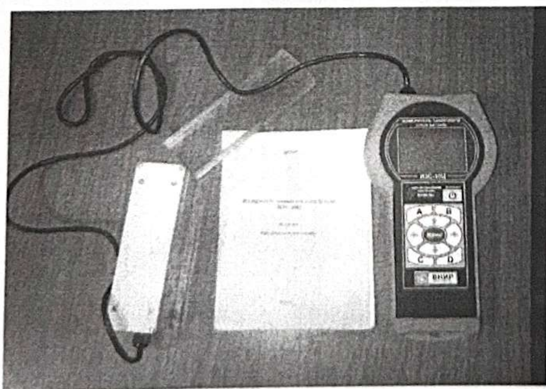
Электронный измеритель защитного слоя бетона «ИЗС-10Ц»
